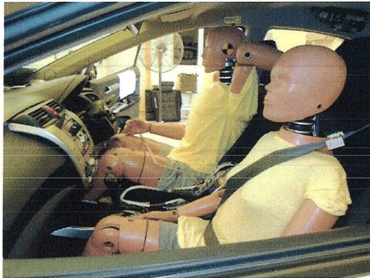
PC-3での実車試験に搭載されるジャスティ製ダミー
